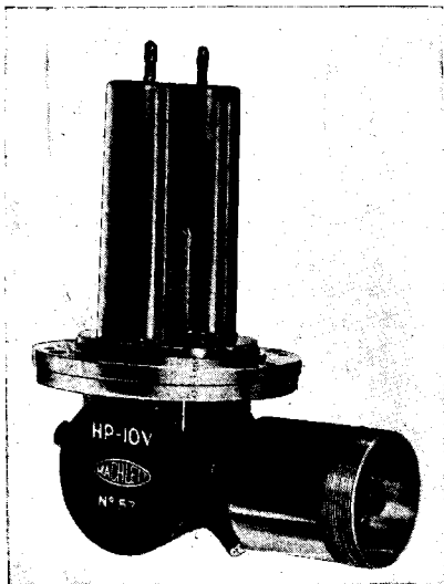
FIG. 19-24.—HP10V magnetron.
